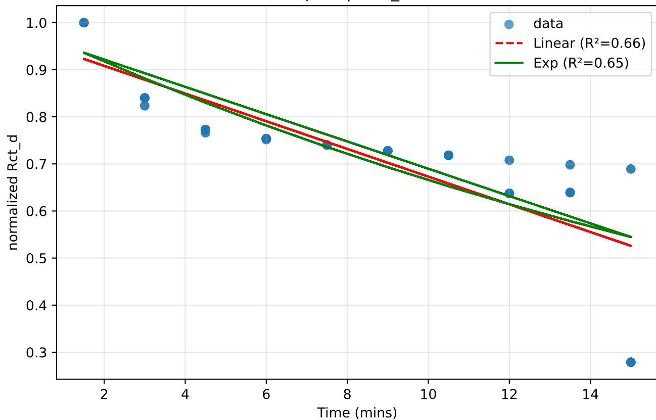
Chip 46 | 1nM_asso
